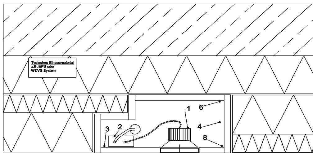
Schnitt Längs / Standard Aufbau für Temperaturmessungen
